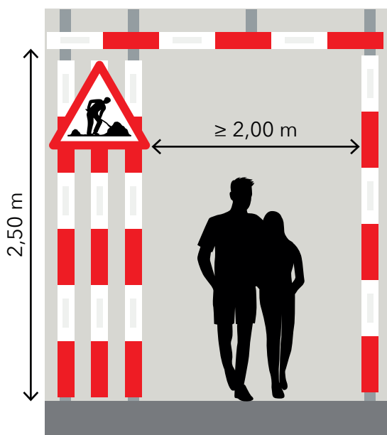
1. Standardbreite \geq 2,00 m
